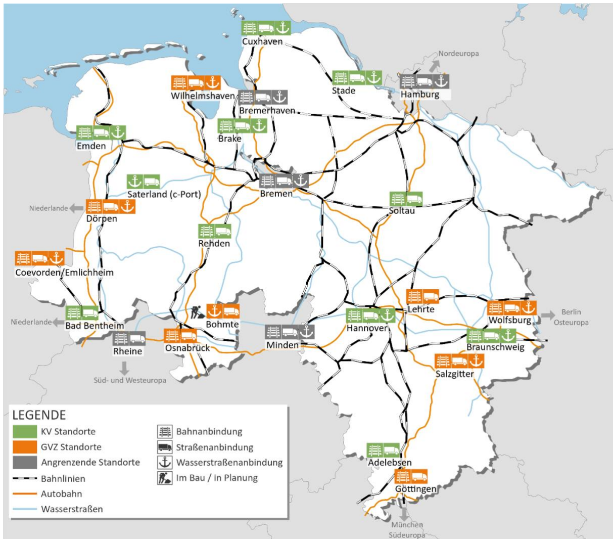
Abbildung 4-6: Terminalkarte Niedersachsen
